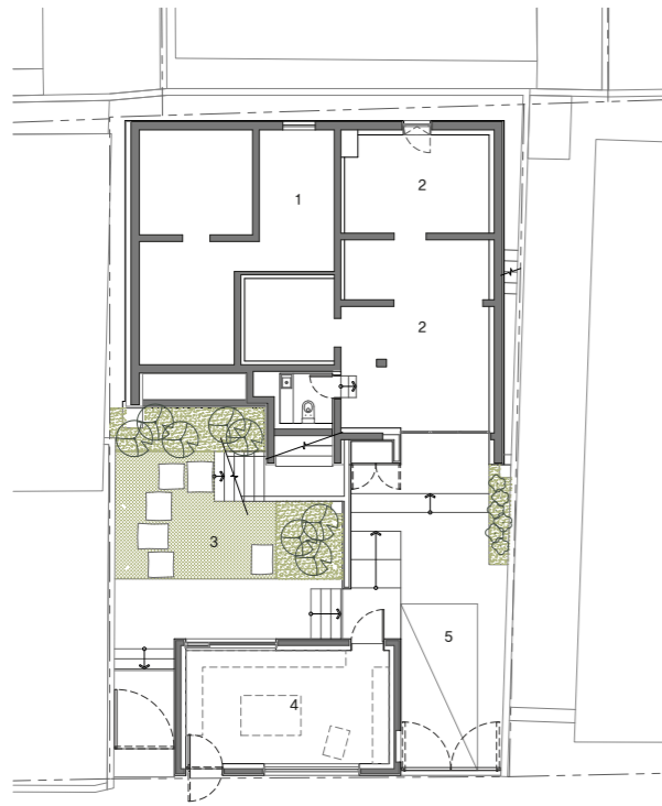
1층 평면도
